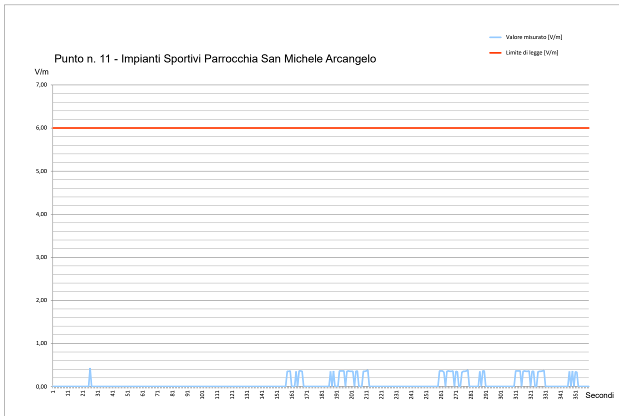
Fig. 37 Grafico Misura di Campo Elettromagnetico a RadioFrequenza – Punto #11
