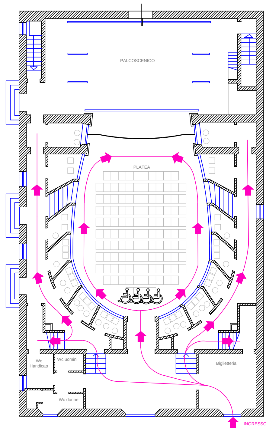
PIANO TERRA (I° ordine palchi)
